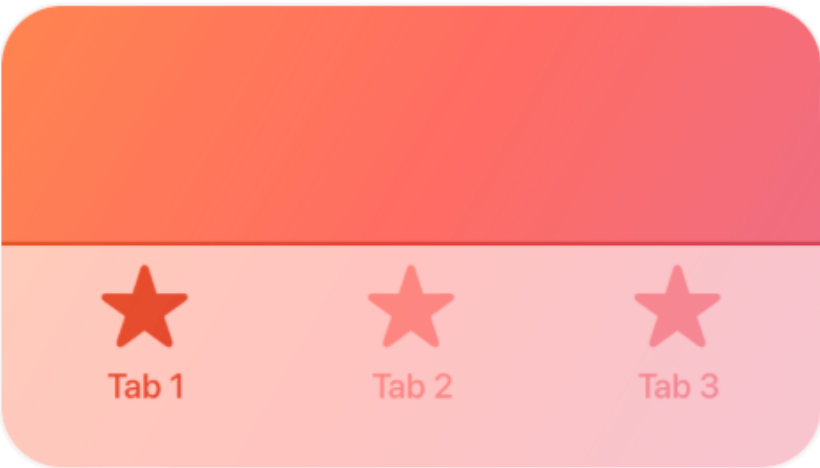
Tab bars
