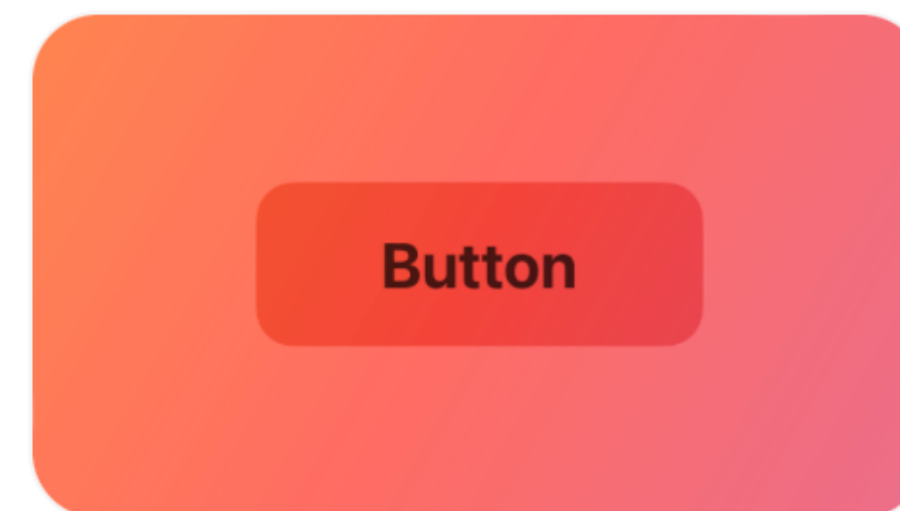
Buttons
