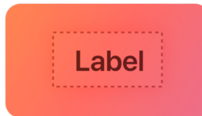
Labels
