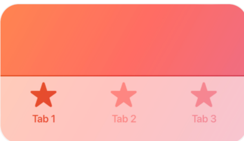
Tab bars
