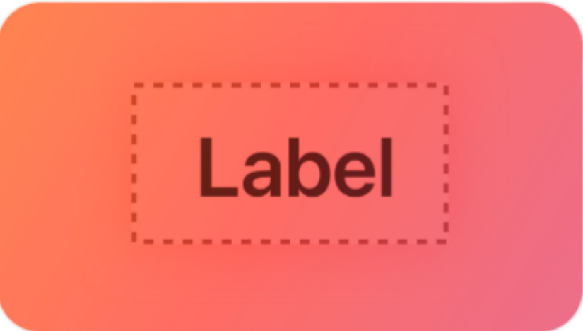
Labels
