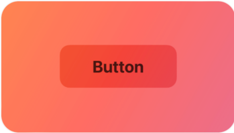
Buttons
