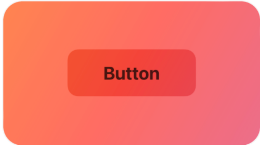
Buttons
