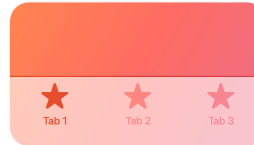
Tab bars
