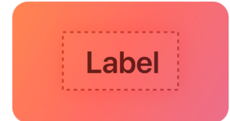
Labels
