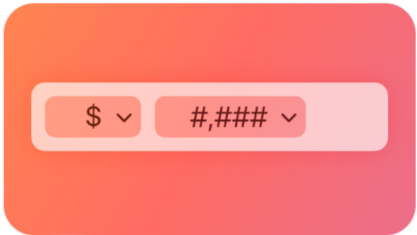
Token fields
