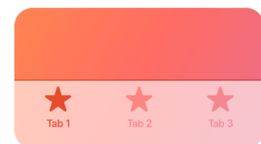
Tab bars
