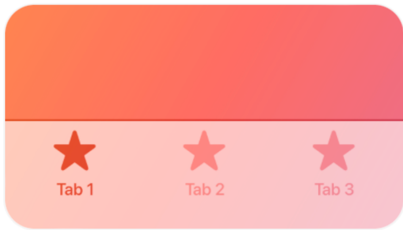
Tab bars
