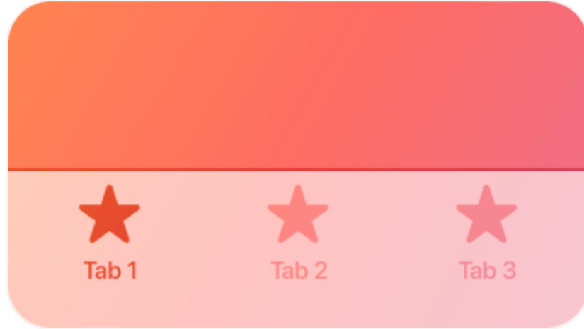
Tab bars
