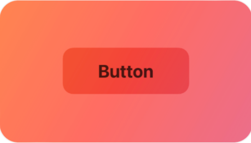
Buttons
