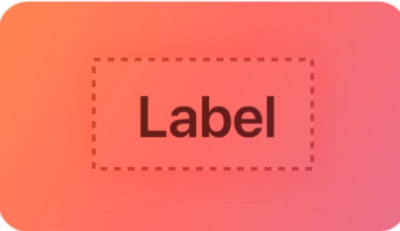
Labels
