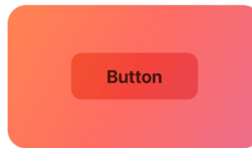
Buttons
