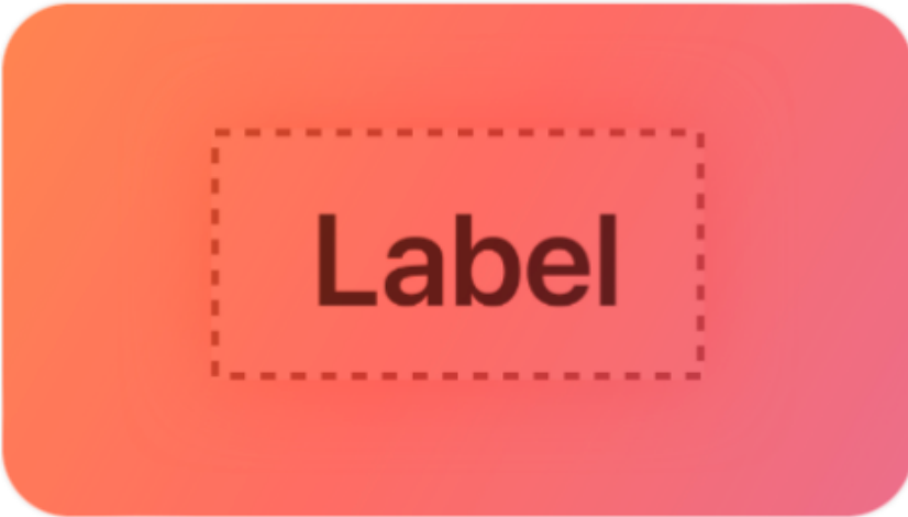
Labels
