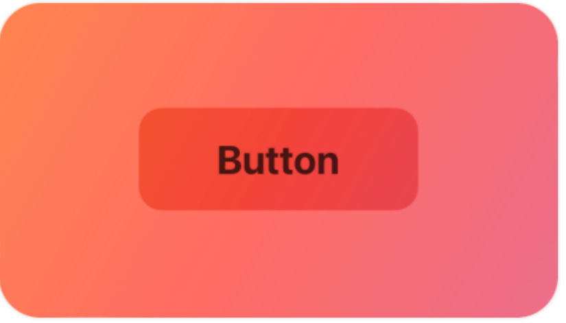
Buttons
